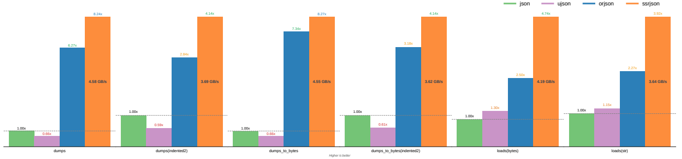
truenull.json
