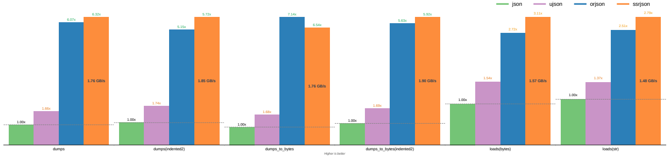
tweet.json
