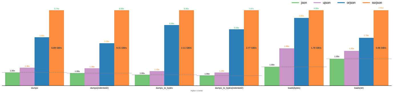
twitter.json
